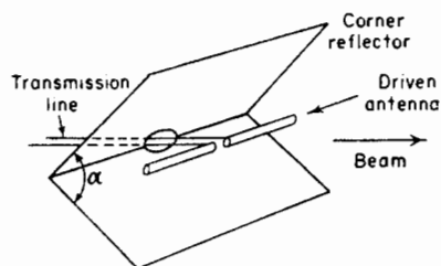
Fig. 12-6. Corner-reflector antenna.
