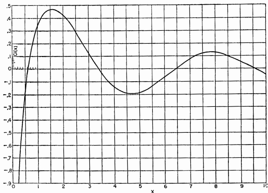
FIG. 5-10. Cosine integral.
