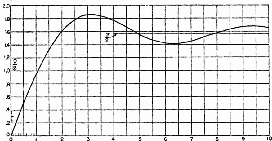
FIG. 5-11. Sine integral.
